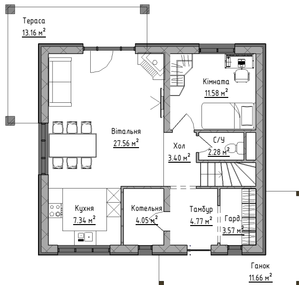
1-й поверх ( 1 : 100 )
