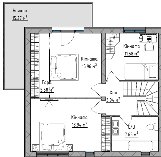
2-й поверх
